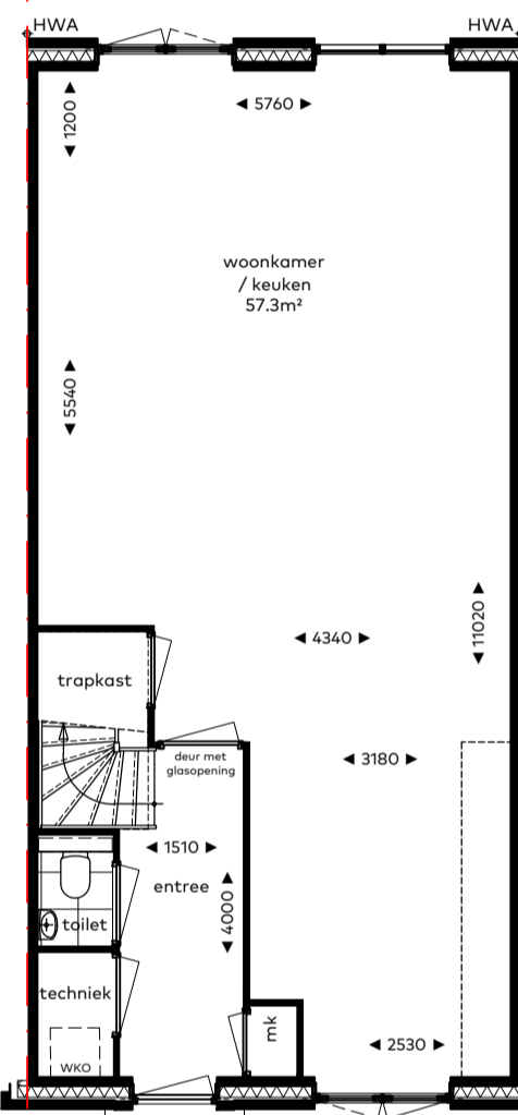
optie E1-01 uitbouw 1,20 m
