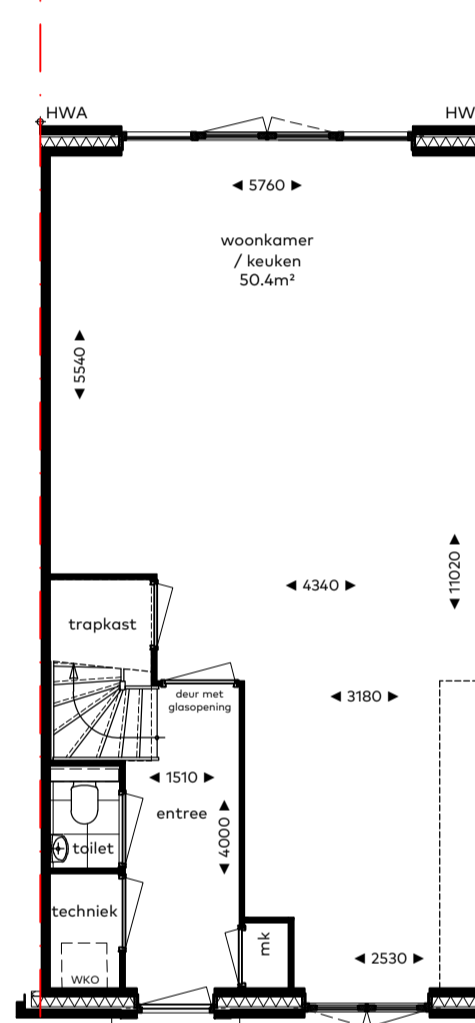
optie E1-03 grote pui achtergevel
