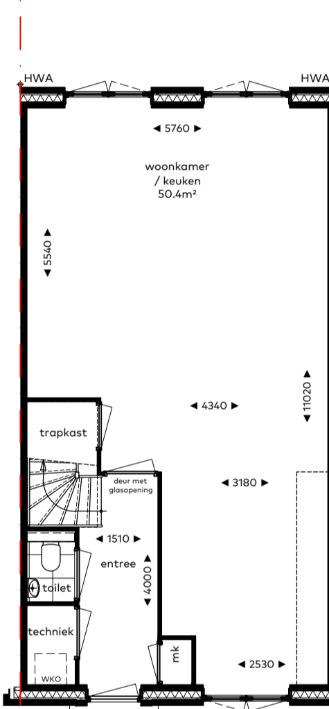
optie E1-02 extra dubbele deur achtergevel
