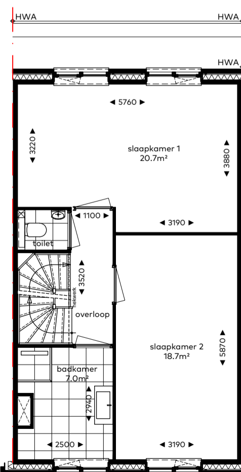
optie E1-05 samenvoegen van slaapkamer 1 en 3
