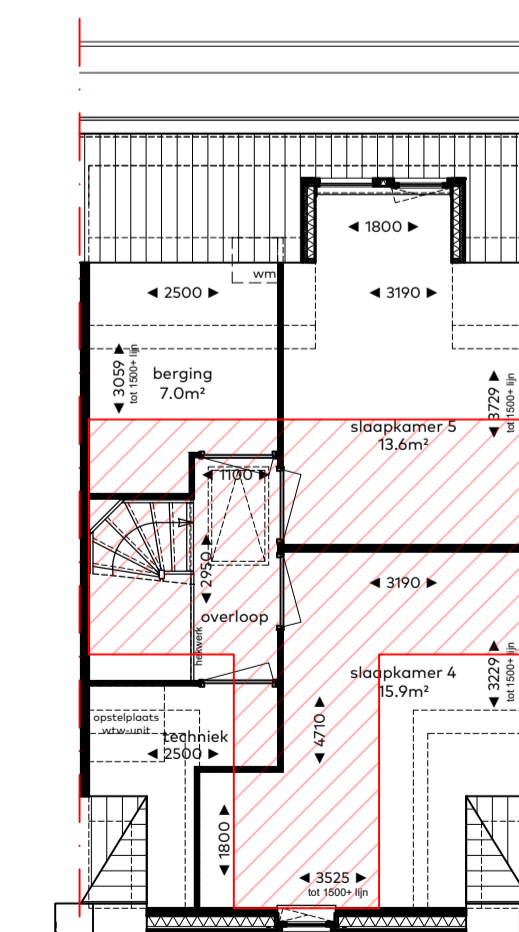
optie E1-10 vloering
