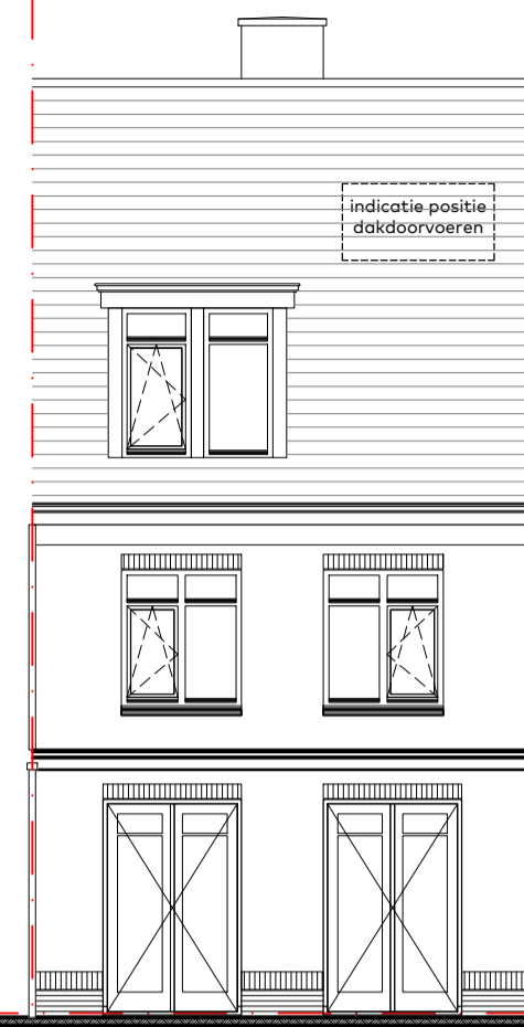
optie E1-02 extra dubbele deur achtergevel
