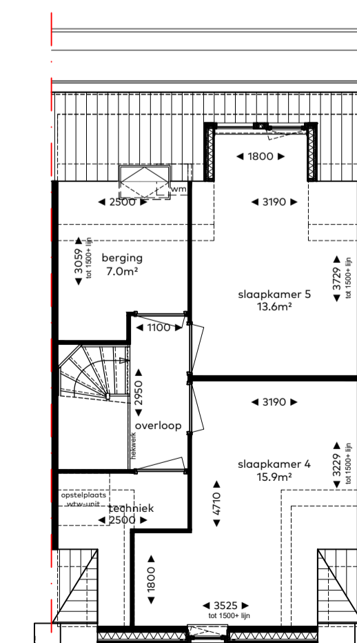
optie E1-09 dakraam achterzijde
