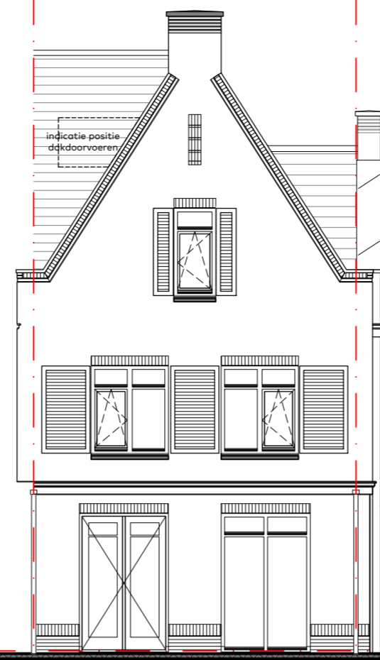
optie E2-08 extra luiken
