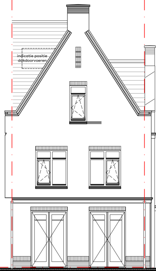
optie E2-02 extra dubbele deur achtergevel
