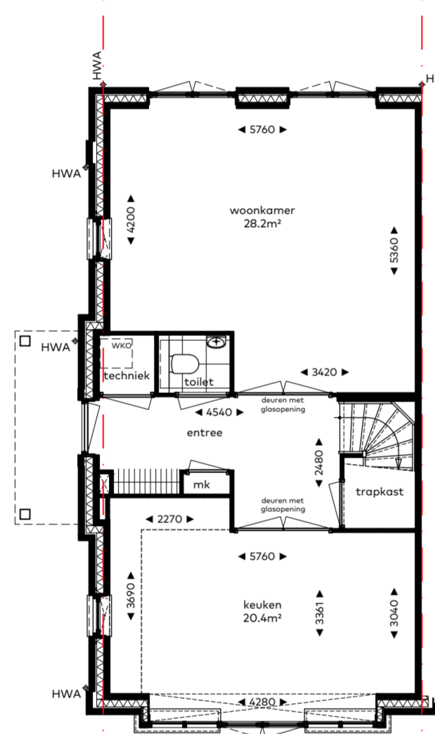
optie E2-02 extra dubbele deur achtergevel
