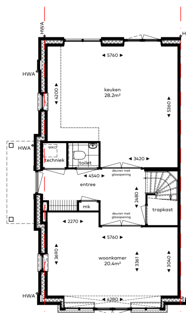
optie E2-04 keuken achtergevel
