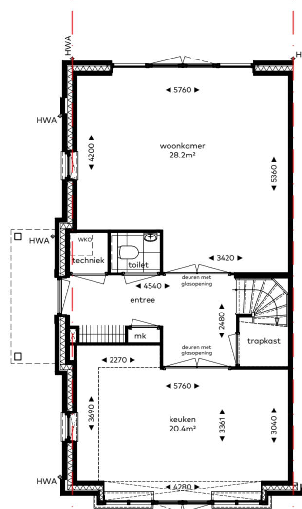
optie E2-03 grote pui achtergevel
