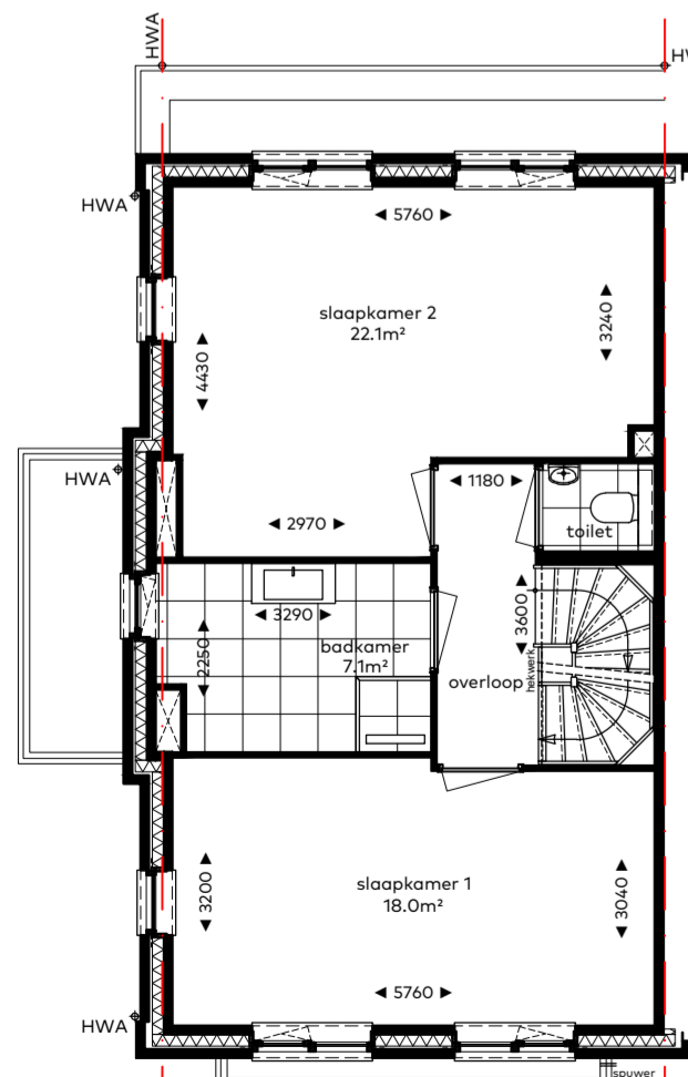
optie E2-05 samenvoegen van slaapkamer 2 en 3
