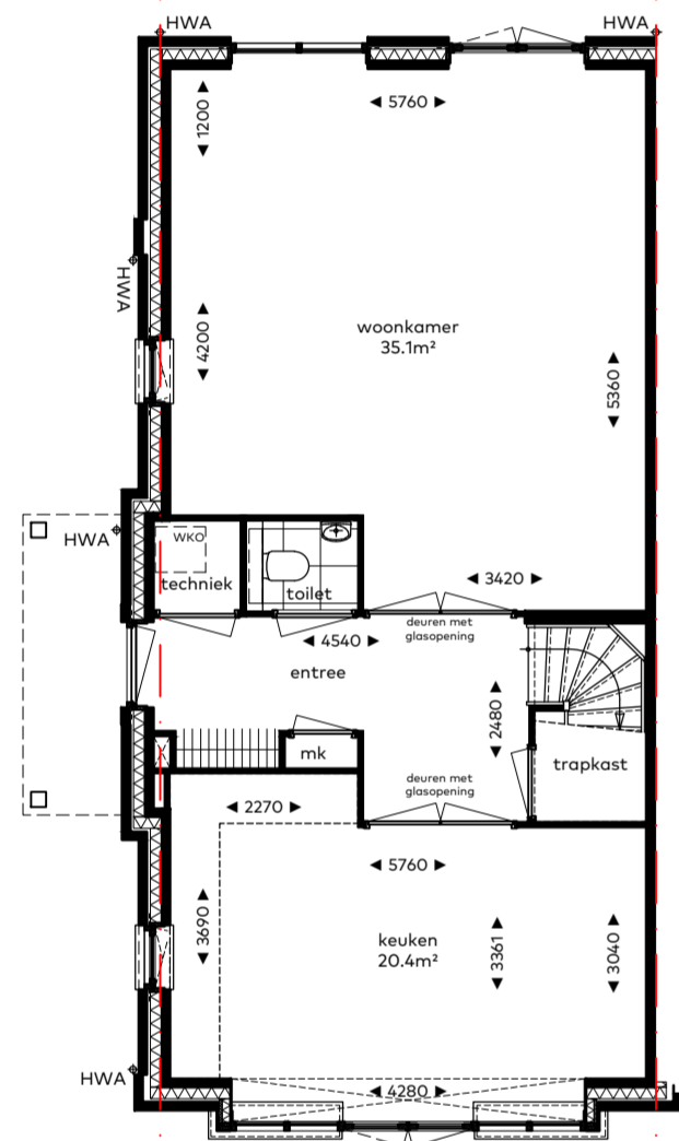
optie E2-01 uitbouw 1,20 m
