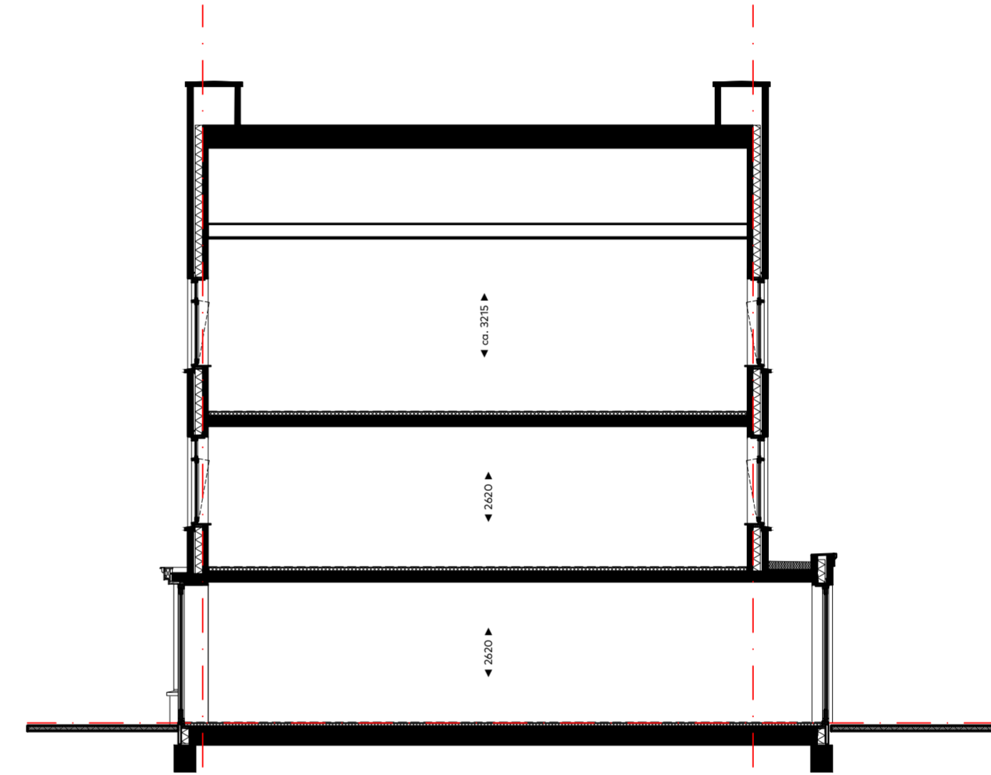
optie E2-07 vloering
