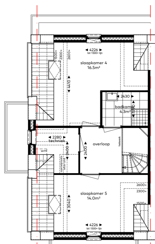
optie E2-06 extra badkamer op zolder
