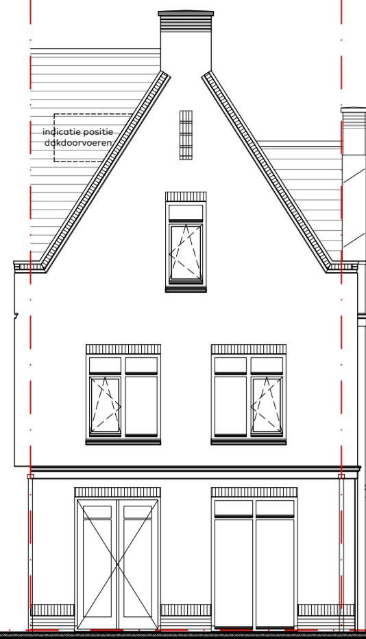
optie E2-01 uitbouw 1,20 m
