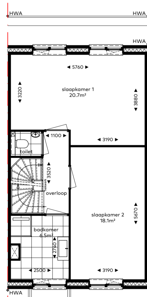
optie E-05 samenvoegen van slaapkamer 1 en 3
