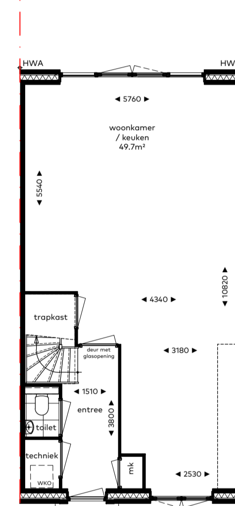
optie E-03 grote pui achtergevel
