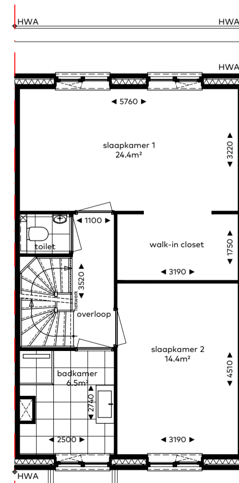
optie E-06 samenvoegen van slaapkamer 1 en 3 + walk-in closet
