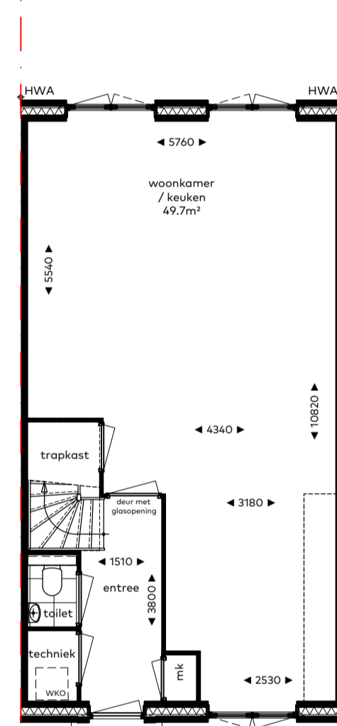
optie E-02 extra dubbele deur achtergevel
